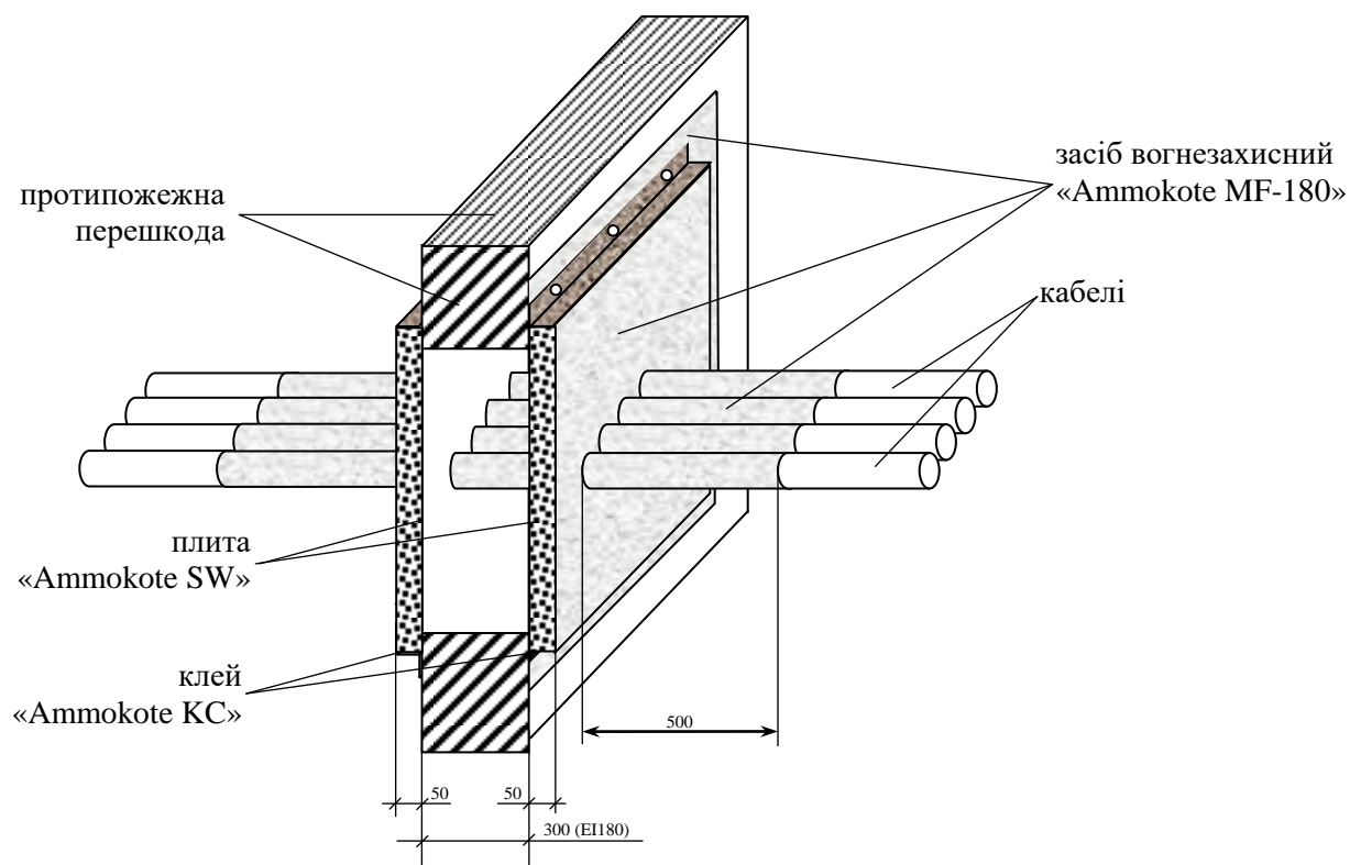
Рис. 2 – Збірна система конструктивного вогнезахисту «Ammokote SCS-K»
